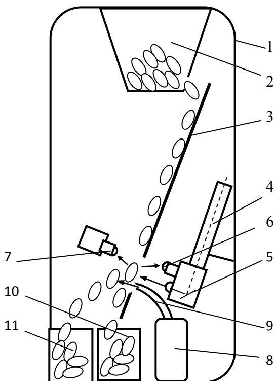
Рис.1. Лазерный сканирующий сепаратор семян для селекции
